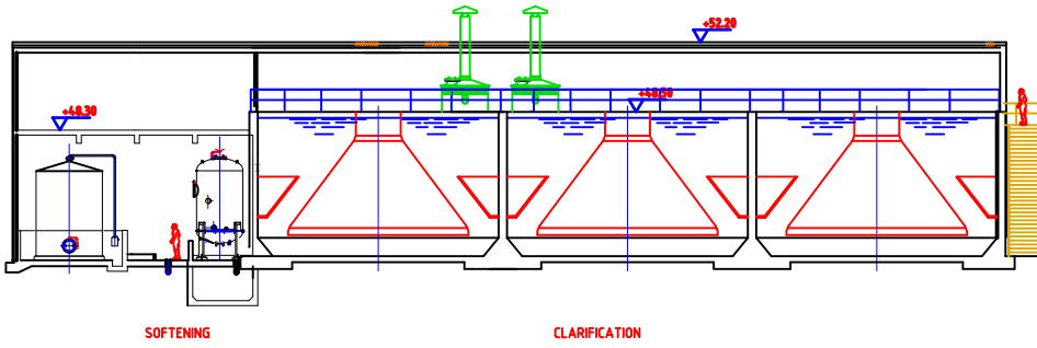
A-A
