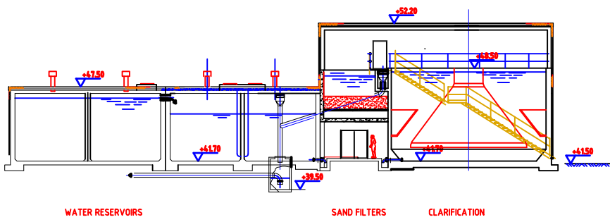
C-C
