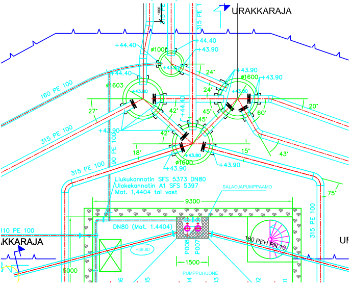
TULOCAIVOT TASO 43.800 (1:50)
