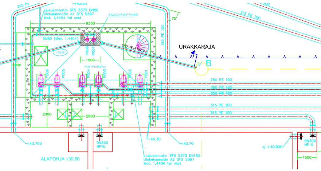
PUMPPAAMO TASO 39.800 (1:50)
